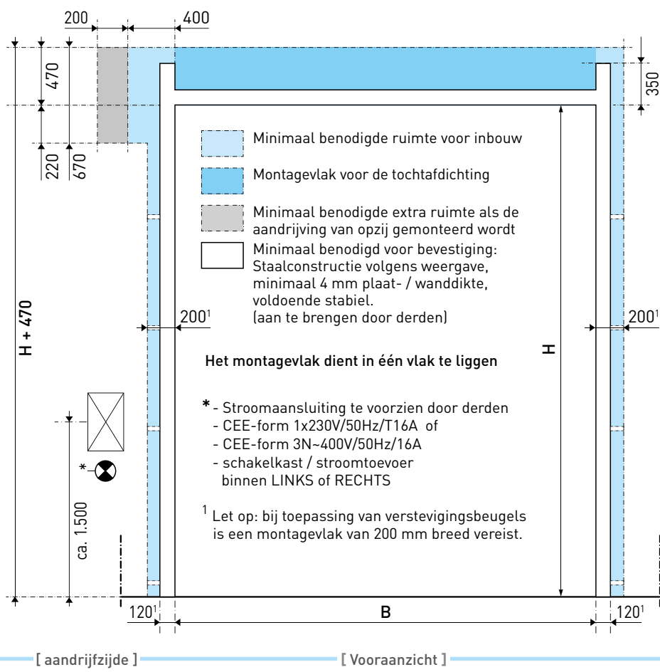
[ aandrijfszijde ]
